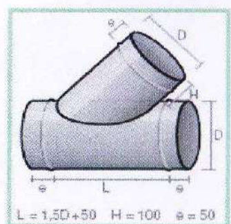
TV SIMPLE A 45°
