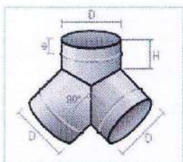
* PANTALÓN SIMPLE 45° YV
