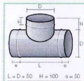
TC SIMPLE A 90°
