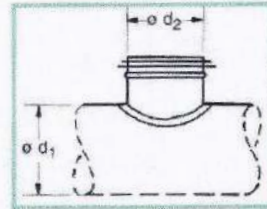
INJERTO 90° C/JUNTA PSL
